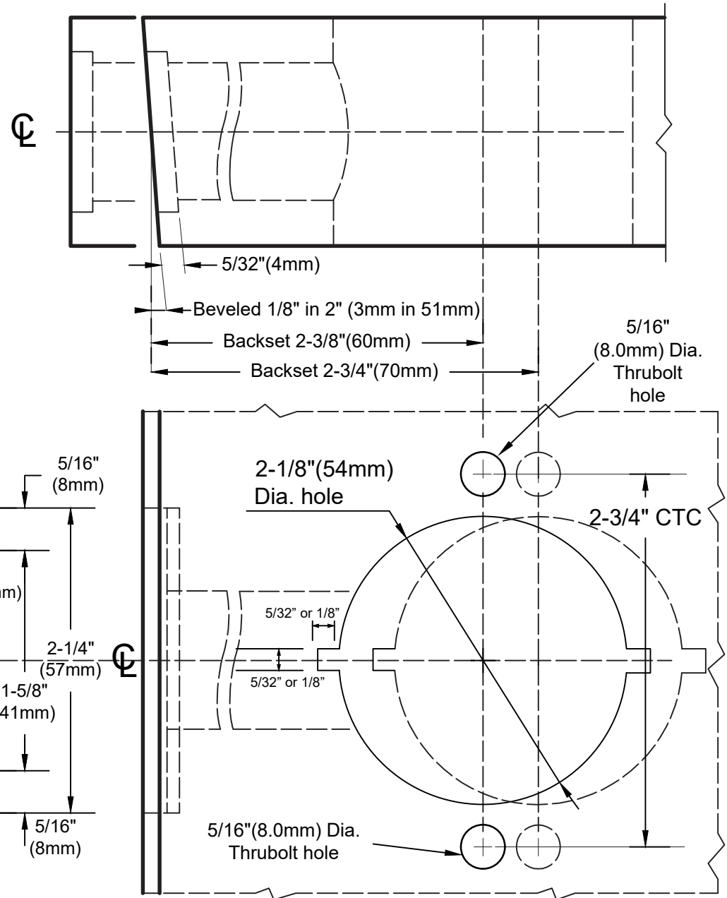
Optional 2-3/8" Latch
